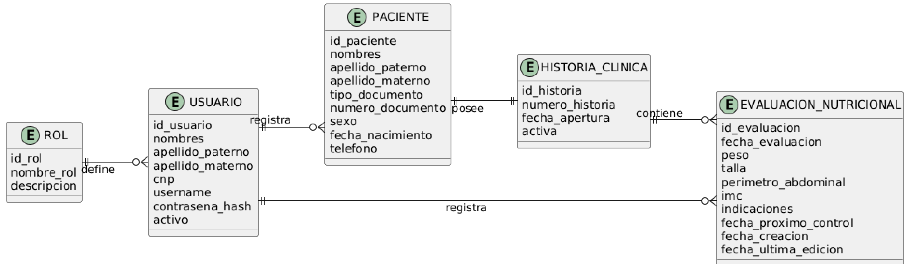
Sistema de Control de Peso — SISCOP Modelo Entidad-Relación
